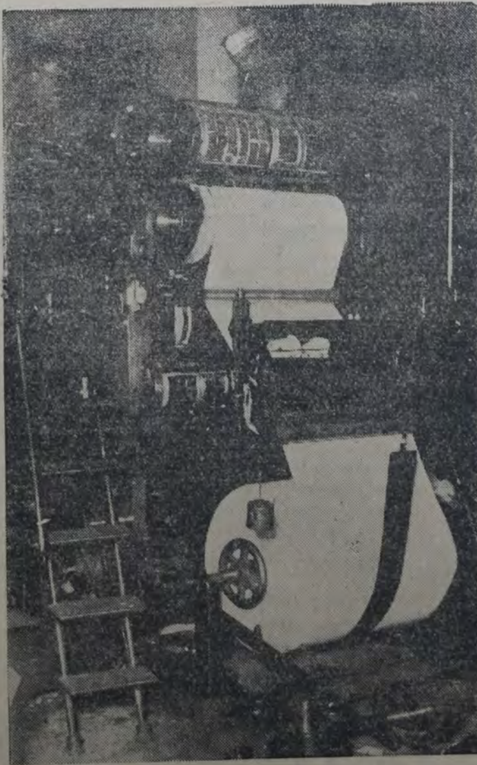
8. — LA "ROTATIVA" CON UNA DE LAS "BOBINAS" DE PAPEL LISTA para funcionar. Los "clichés", de forma semicilíndrica y que corresponden a cada página, se colocan en "los tambores" que, mediante complicados engranajes al girar ponen en contacto el papel y los "clichés" debidamente entintados por los "rodillos". Así preparada la máquina comienza a funcionar, y arroja ejemplares doblados y listos para salir a la venta, a razón de más de quince mil por hora, en la forma que puede verse en nuestro grabado de la primera página.
