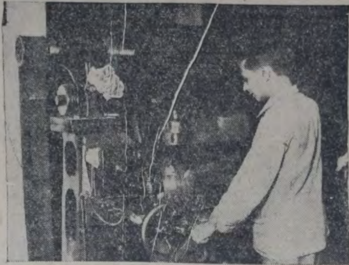
7. — LA MAQUINA FRESADORA SE UTILIZA PARA LIMPIAR EL "CLICHÉ" recién fundido. Esta operación se completa en seguida con pequeños formones.
